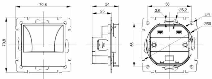
Рисунок 1 – Габаритные размеры подсветки
